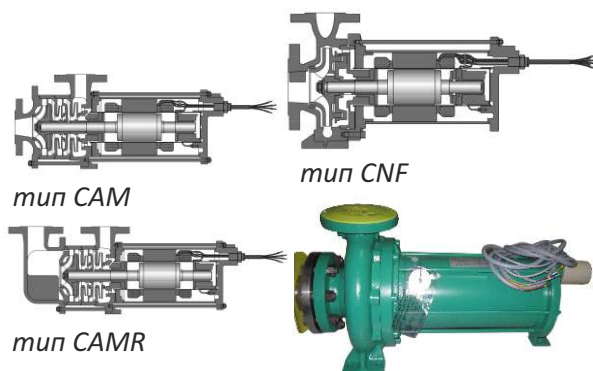
Насос CNF 50-200
